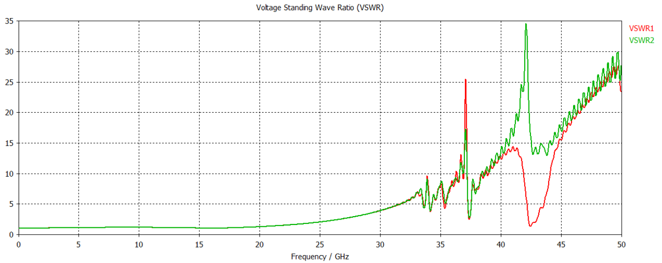
Fig.5 : VSWR
