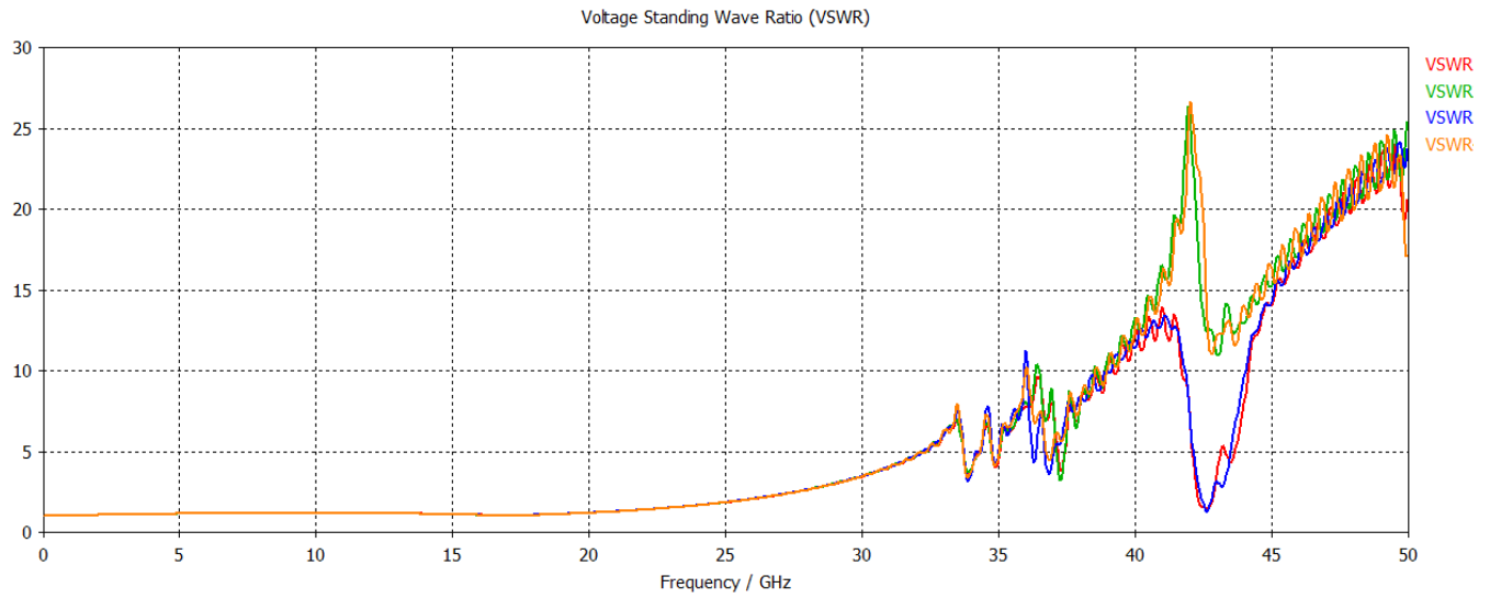
Fig.5 : VSWR
