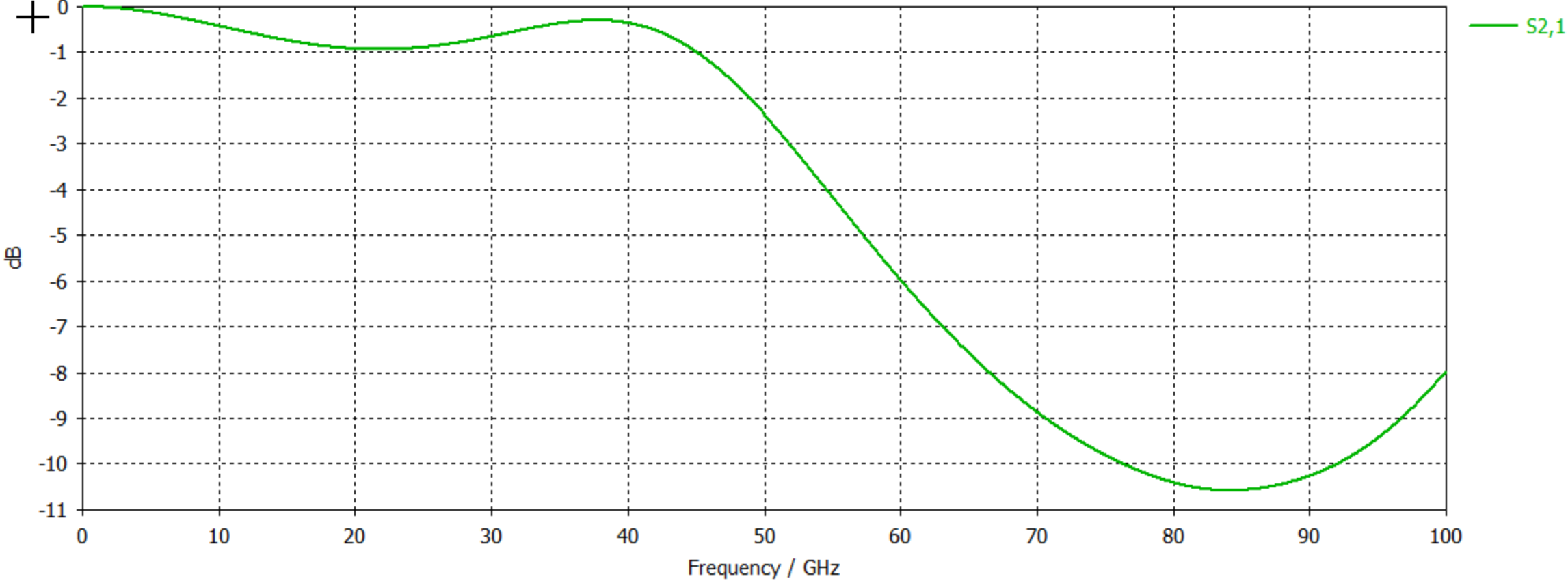
S-Parameters [Magnitude]
